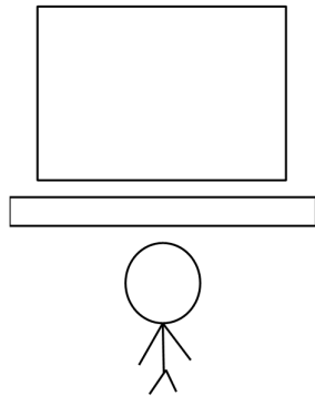
Fig 1.4: Single-User OS
