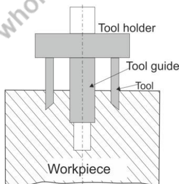
Fig. 5.40: Trepanning
